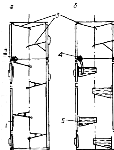
б) экранный
