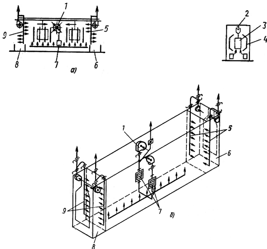
а) схема конструкции; б) схема движения воздуха
