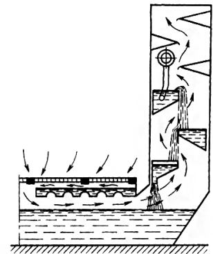
в) экранный
