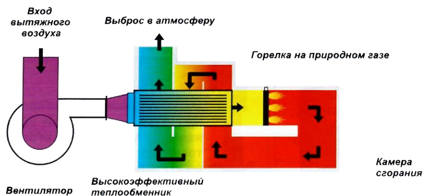
Рисунок 25 — Диаграмма воздушного потока термического рекуперативного окислителя [55]
