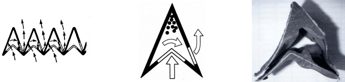
Рисунок 7 — Картонный инерционный фильтр [57]
