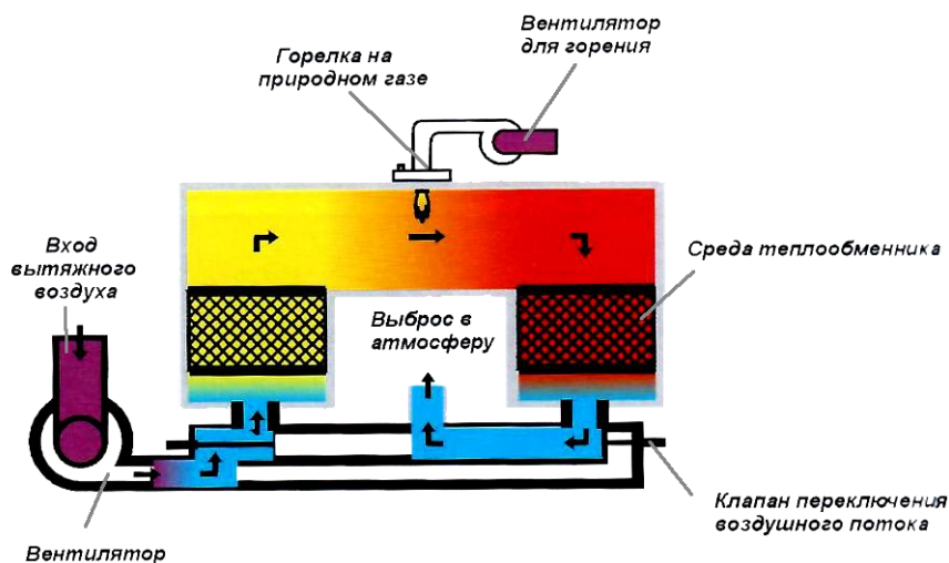
Рисунок 26 — Диаграмма воздушного потока термического регенеративного окислителя [55]
