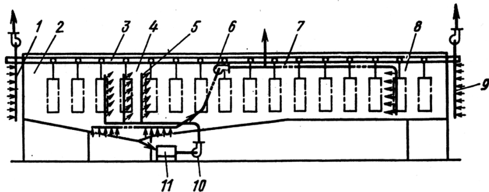
Рисунок 18 — Оборудование для нанесения окупанием [66]
