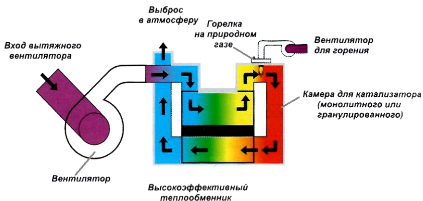
Рисунок 27 — Диаграмма воздушного потока каталитического окислителя [55]
