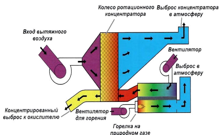
Рисунок 28 — Диаграмма воздушного потока системы ротационного концентратора [55]
