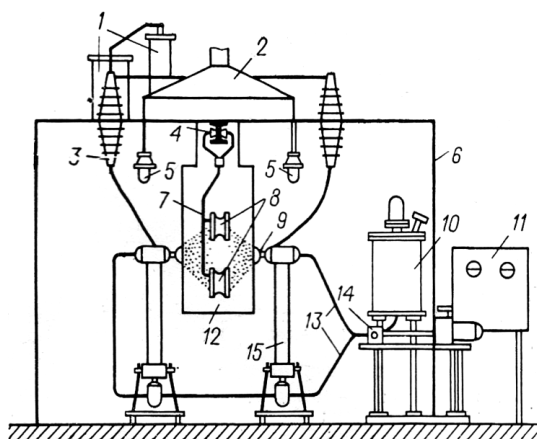
Рисунок 16 — Оборудование при окрашивании безвоздушным распылением [62]
