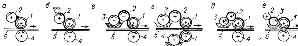
Рисунок 20 — Оборудование для нанесения электроосаждением [62]
