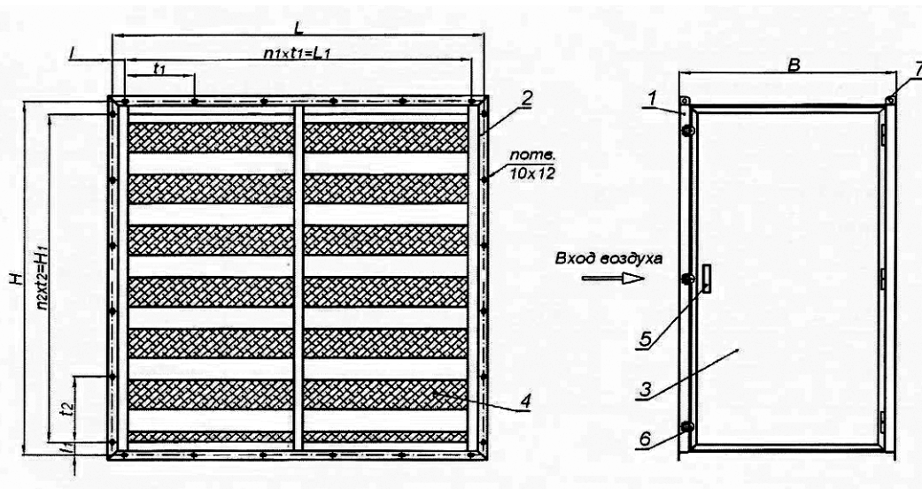
1 — корпус; 2 — фланец; 4 — фильтрующие ячейки; 5 — ручка; 6 — прижим; 7 — проушины для строповки
